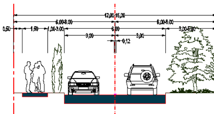
Diófa utca, Temető utca környezetében rögzített kiszolgáló út kialakítása
