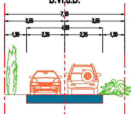
Lakó-kiszolgáló út /szűkületben/ B.VI.d.D.
